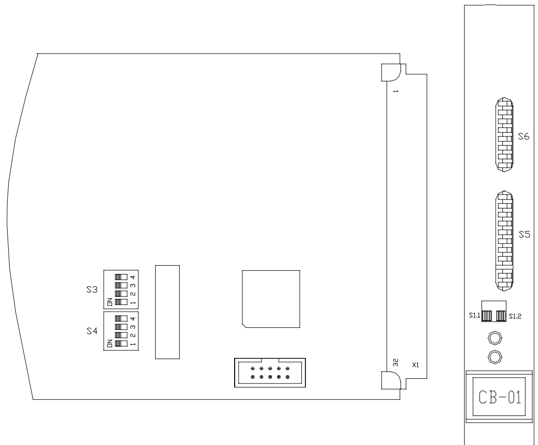
Рис. 1. Плата СВ-01. Схема расположения эксплуатационных переключателей.
