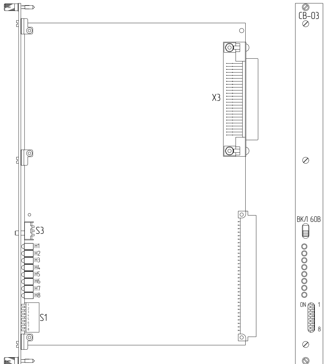
Рисунок 1. Плата СВ-03. Схема расположения эксплуатационных переключателей и разъемов.
